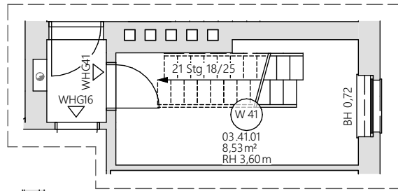
Grundriss 3.OG
